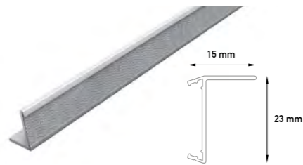
Pritrdilni trak kavelj - Ježek / Hook tape
