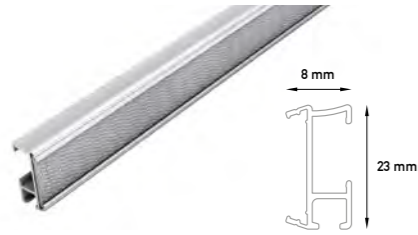
Pritrdilni trak kavelj - Ježek / Hook tape
